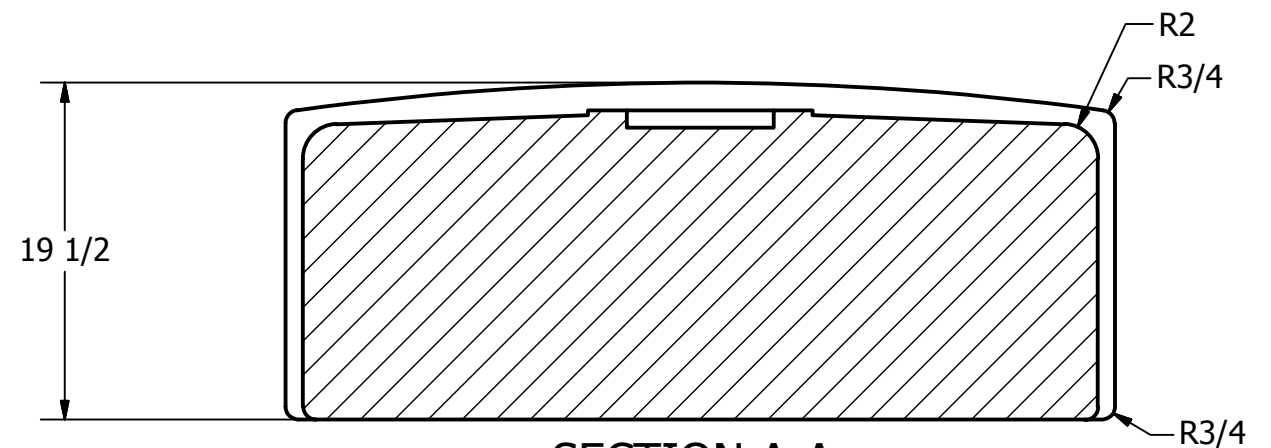
SECTION A-A
